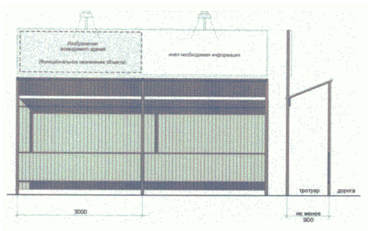
Тип 1.2. Строительное ограждение с навесом и защитным ограждением
